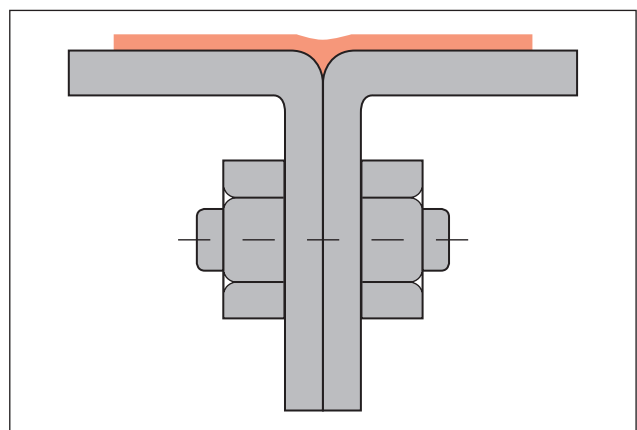
Flächen-Abdichtung
