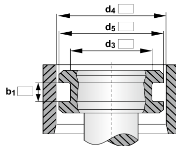
Kolbendichtung
