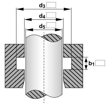
Stangendichtung
